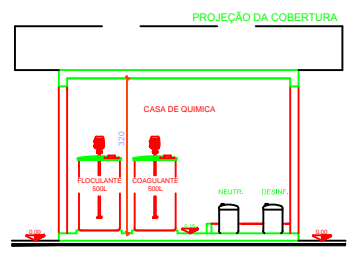
CORTES 01 ESCALA 1/50
