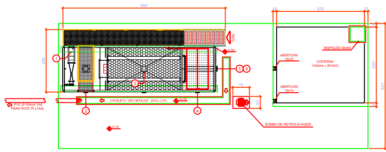
PLANTA BAIXA ESCALA 1/50
