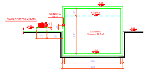
DETALHE DA CISTERNA ESCALA 1/50
