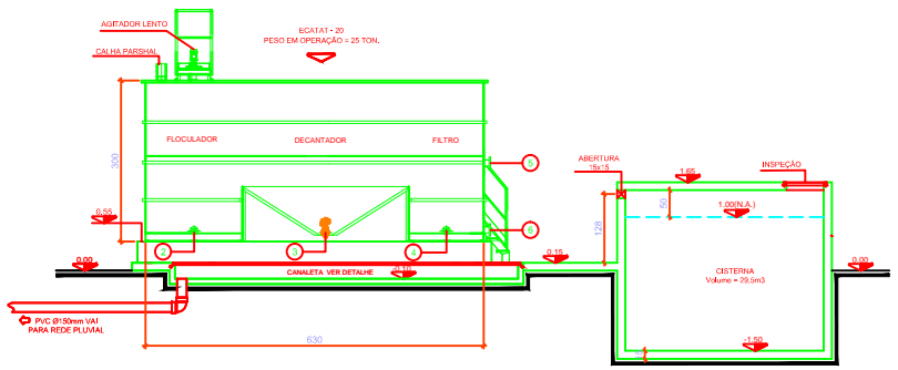
PERFIL LONGITUDINAL ESCALA 1/50
