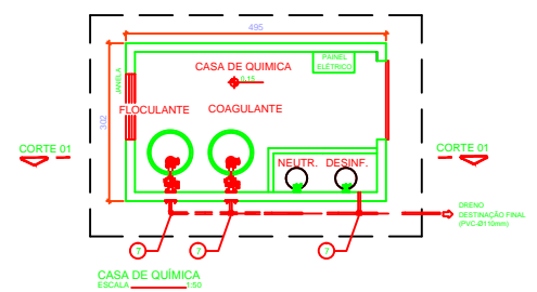
CASA DE QUÍMICA ESCALA 1/50
