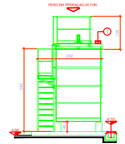
PERFIL LATERAL DA ESTAÇÃO DE TRATAMENTO ESCALA 1/50
